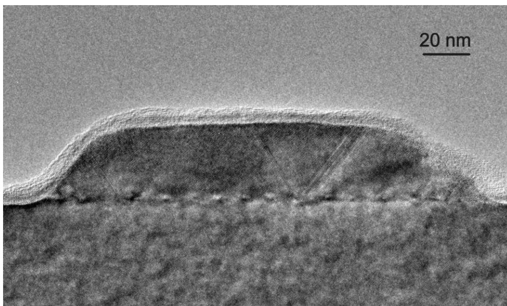
Obrázok 1. Priečny rez InMnAs kvantovou bodkou pripravený pomocou vysoko rozlišovacieho elektrónového mikroskopu Titan 320 keV
